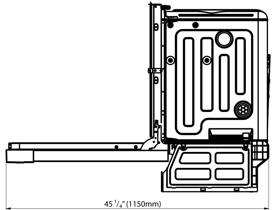
Door Swing
